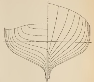
Fig. 4. Posición de las costillas de proa y de popa del yacht Ostsee
